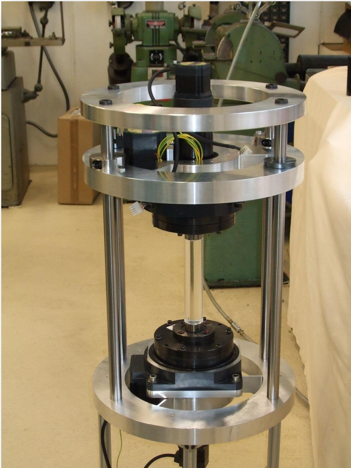
Machine de traction, compression et torsion pour tomographe.
