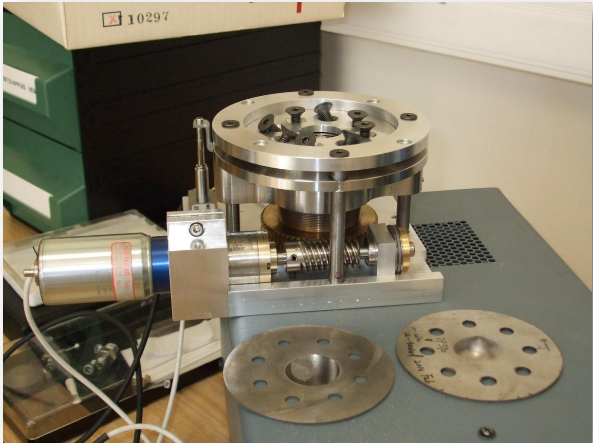
Machine de poinçonnement sur des échantillons métallique
